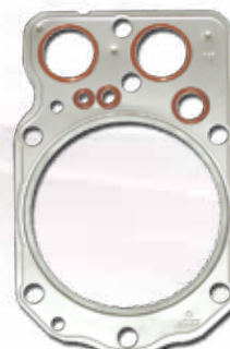
《6D22/6D22-T/6D24-T》 (5-0 RING)
